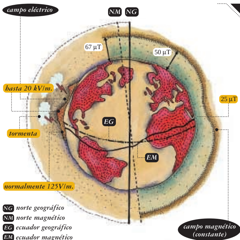
Figura 8. Campo estático natural de la tierra.
