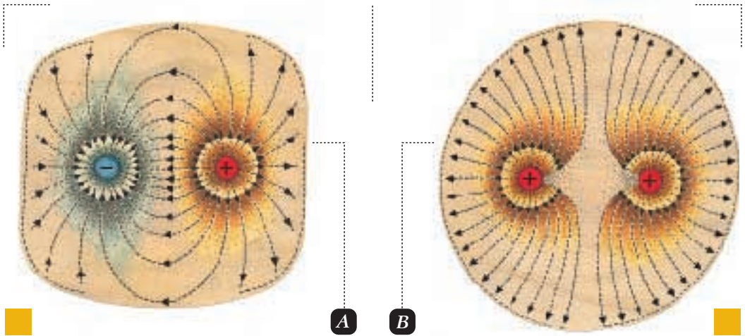
Figura 4. A) Líneas de campo eléctrico entre dos cargas iguales y de signo opuesto.
