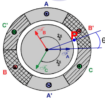
Sistema trifásico
